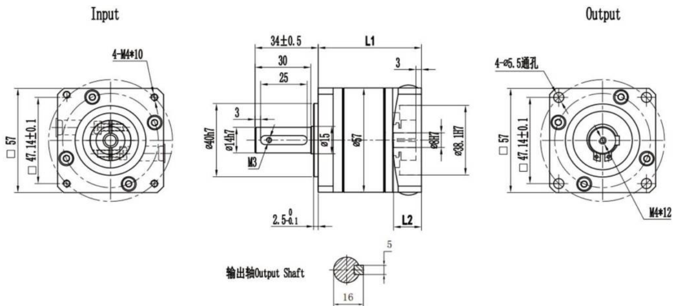
WLF57-50 wymiary
